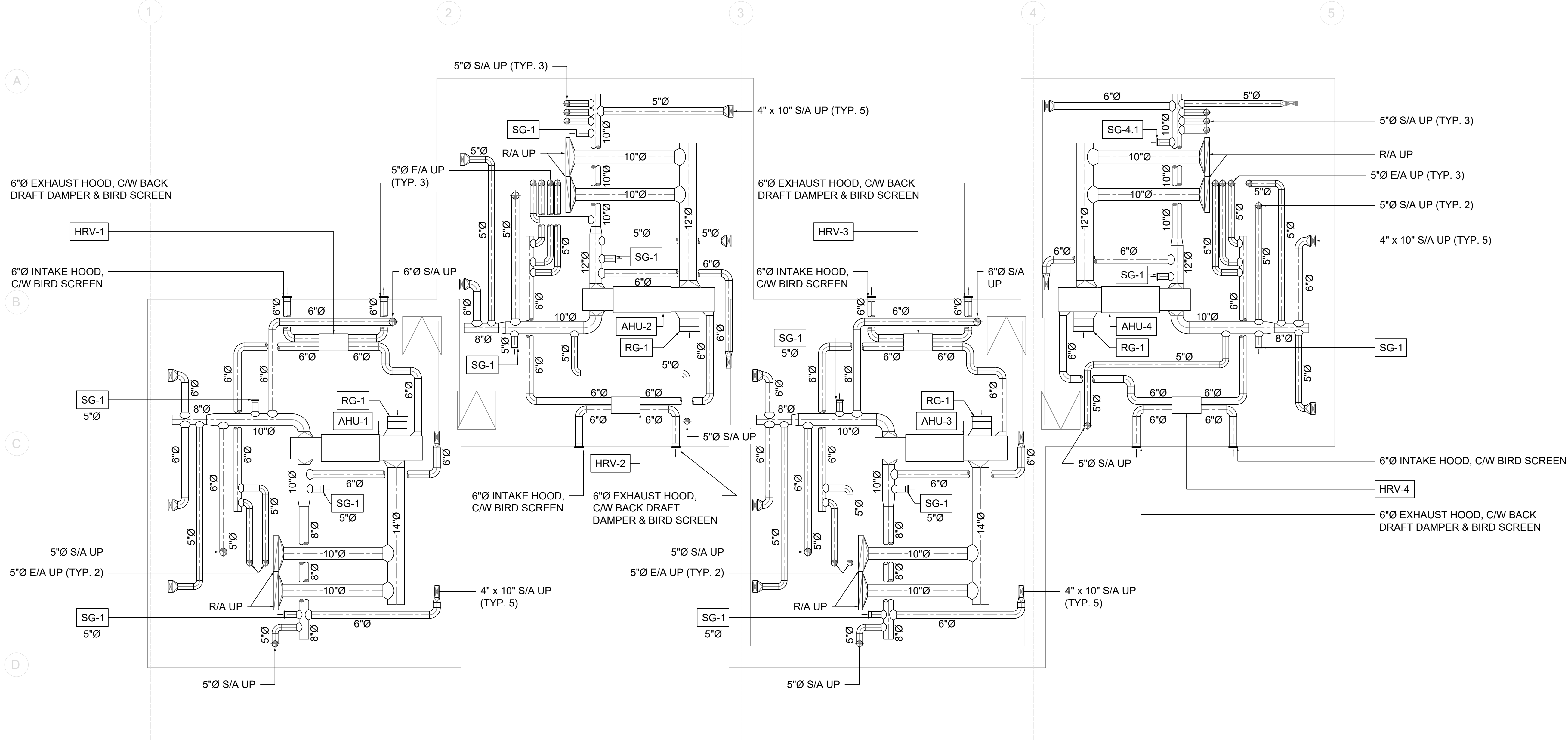
M0 1 CRAWL SPACE PLAN 1/4" : 1'
